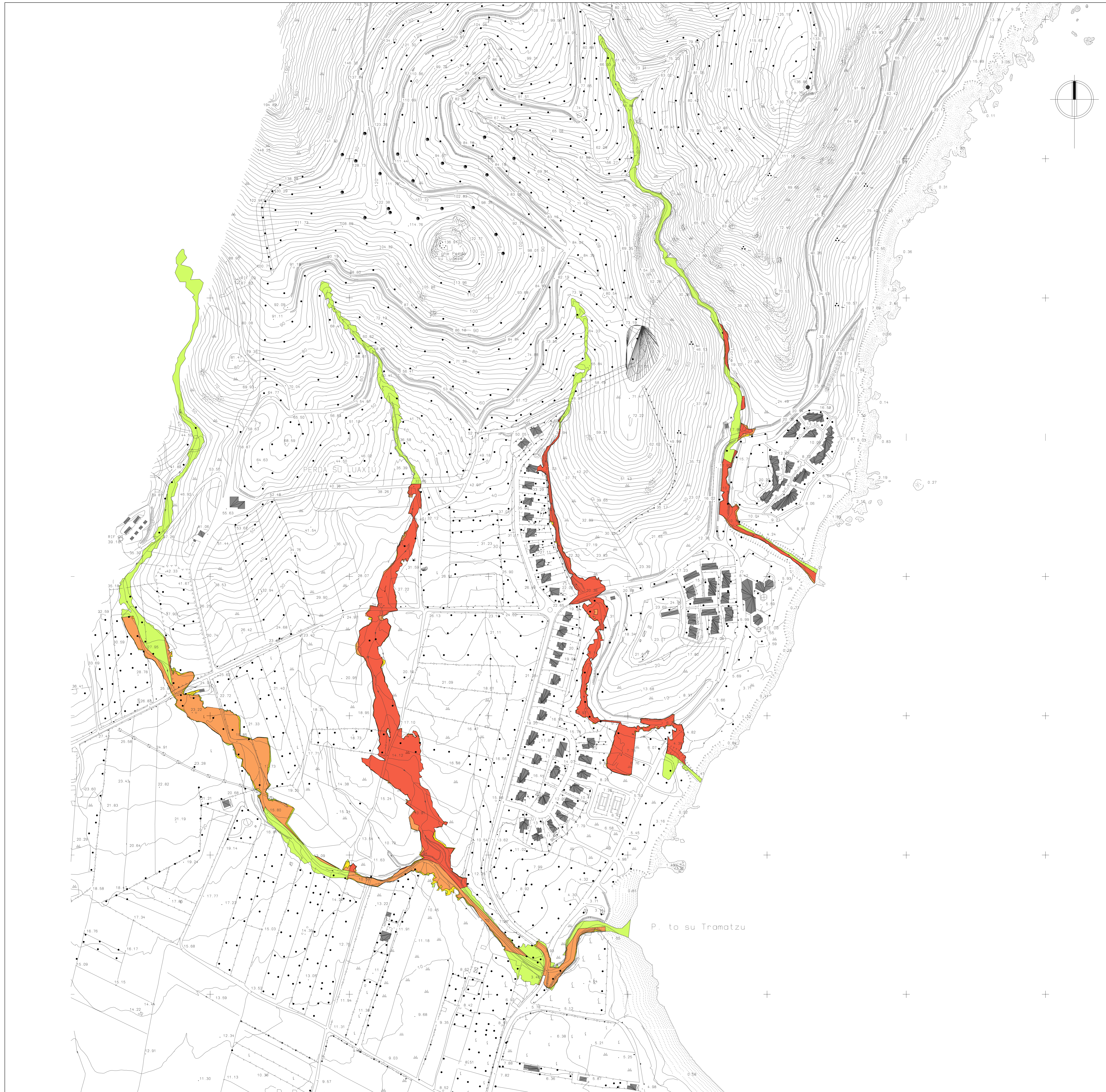
CARTOGRAFIA RISCHIO IDRAULICO ZONA TURISTICA "PORTO SU TRAMATZU" Scala 1:2.000
